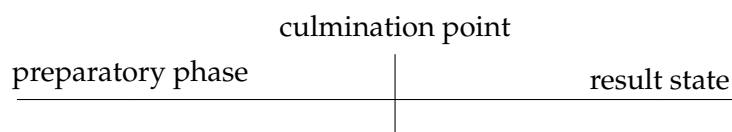
Abb. 4.1: Ereignisnukleus
